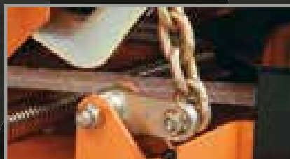
Système de réglage du plateau de coupe sur les quatre côtés, garantissant des réglages aisés pour une tonte régulière.
