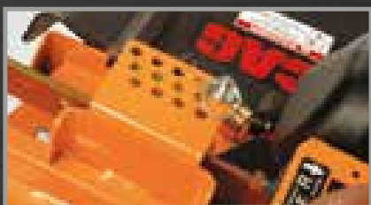
Règlage de la hauteur de coupe aisé de 2,5 à 11,5 cm par palier de 6 mm. En option, le plateau est verrouillable pour le transport.
