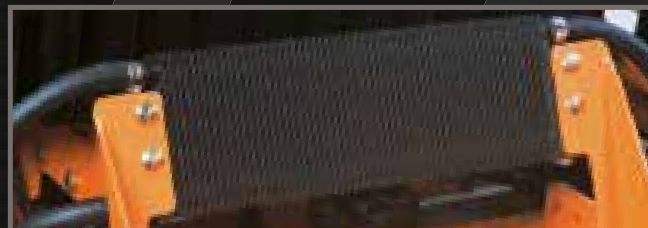
Radiateur d'huile gardant les températures hydrauliques basses pour un fonctionnement efficace, une meilleure fiabilité et une longévité du composant.
